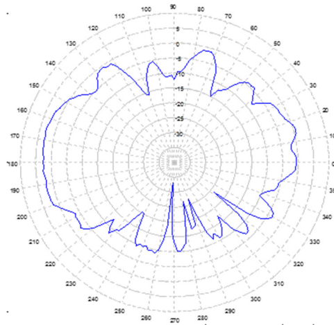
4.95 GHz. ELEVATION
